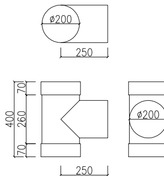
T - KUS (45°,90°)
